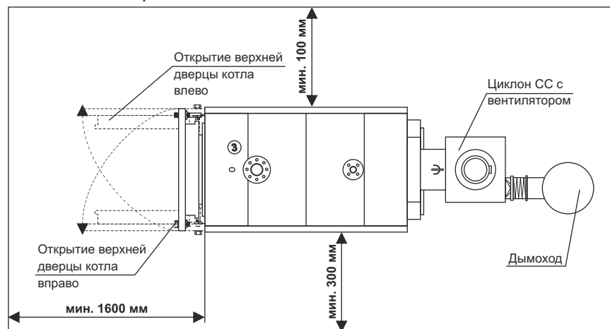
Рис. 1 Минимальное расстояние от стены в котельной
